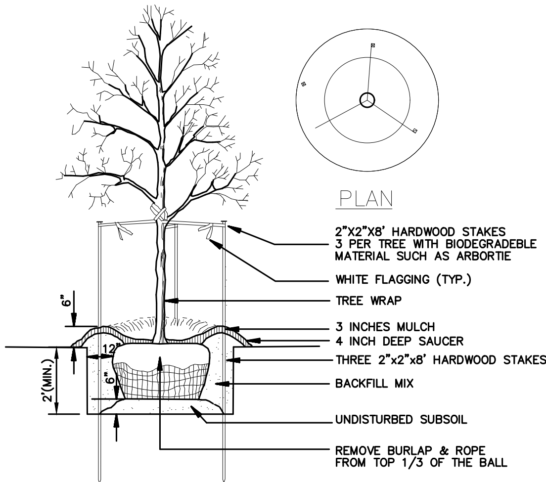
TREE PLANTING N.T.S.
